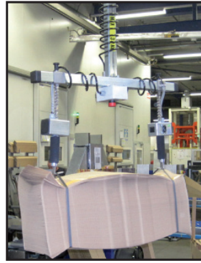
Werkzeug zum Heben von Papiersackbündeln.
