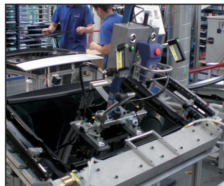
Spezialwerkzeug zum Heben von Autodächern aus Glas.
