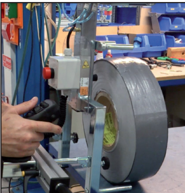
Rollenhandling mit pneumatischem Greifer / Heben von Papierrolle mit justierbarer Joystick-Steuerung.
