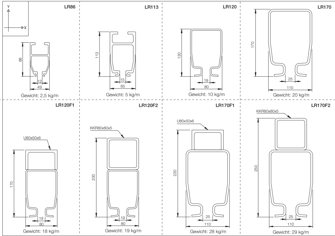
Abmaße: Das gesamte Sortiment der Profile finden Sie in einer Bildreihe auf Seite 2. Aluminiumprofile LR86/LR113, Stahlprofile LR120/LR170, verstärkte Profile LR120F1/F2 und LR170F1/F2.
