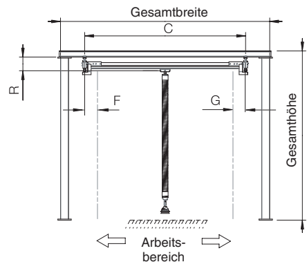
LR120/170 Stahlprofile in einem Niedrigbausystem. SWL bis zu 1.500kg mit verstärkten Profilen. Die freistehende Portal-Befestigungsstruktur ist eine Alternative zur Decken- und Wandaufhängung.
